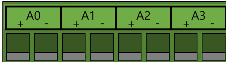
图 1-4 模拟输入端口
