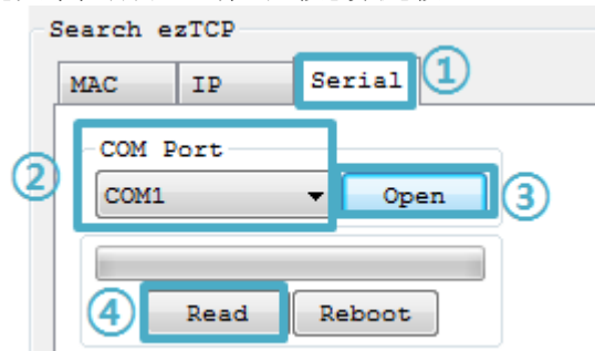
图 2-7 读取串行端口参数
