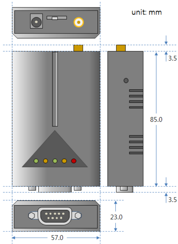
图 1-4 尺寸
