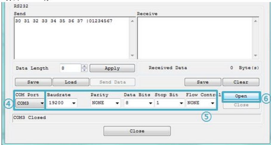
图 2-13 通过串行COM端口打开
