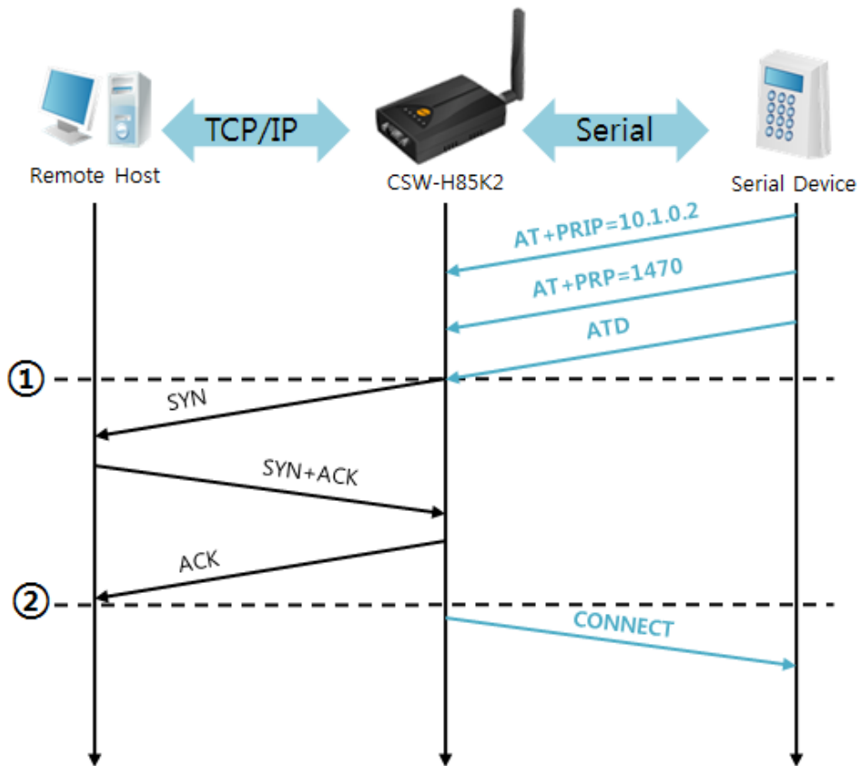
图 5-8 TCP 自动连接
