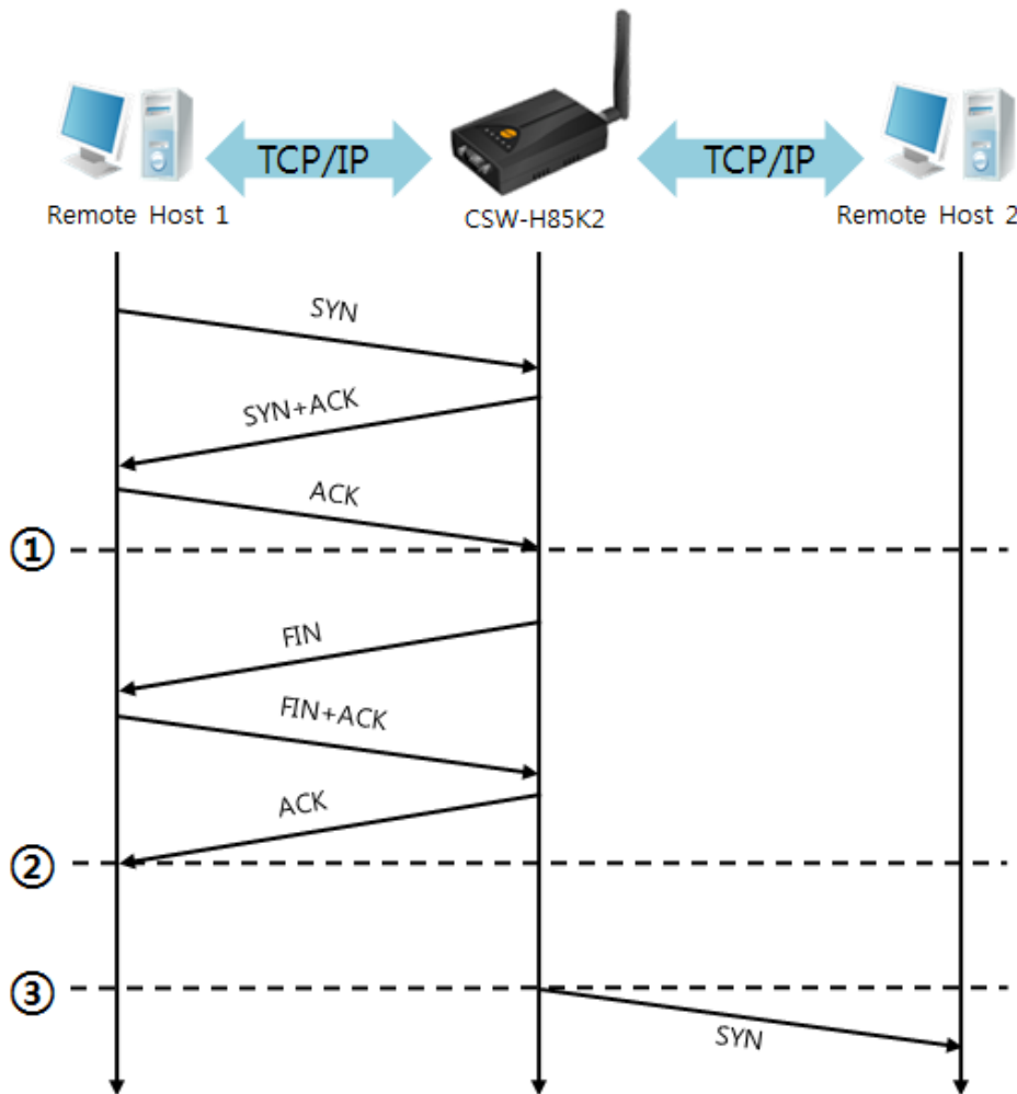
图 5-6 TCP 服务器/客户端模式时
