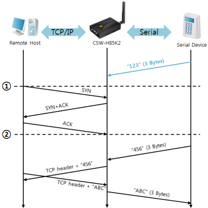
图 5-1 连接前数据代谢大小为0的情况
