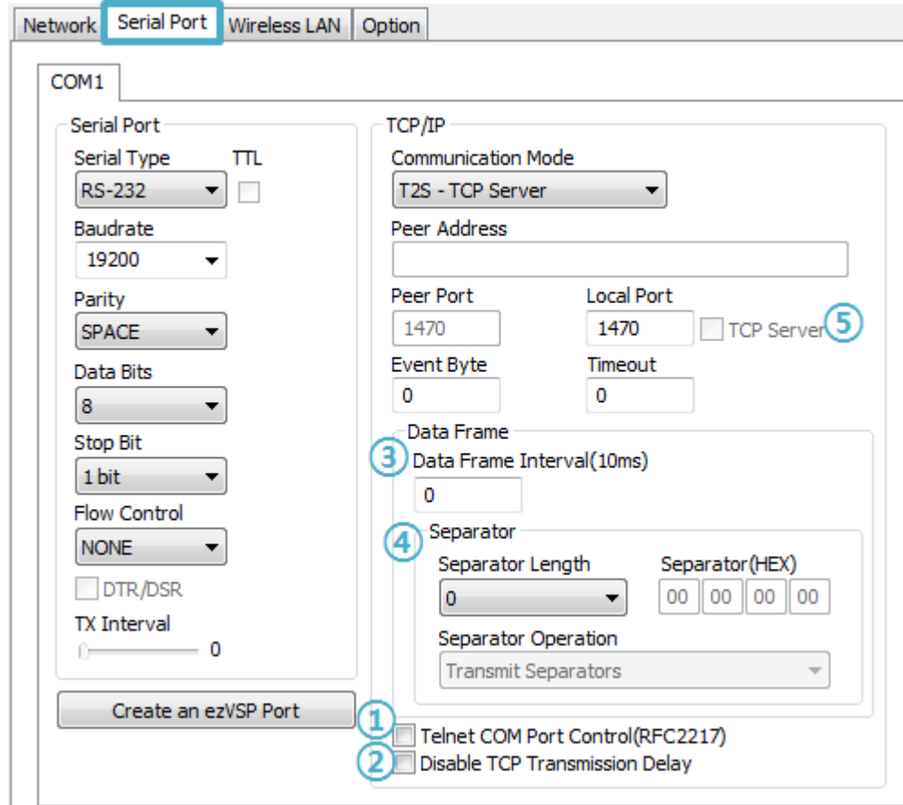
图 7-7 串行端口的功能
