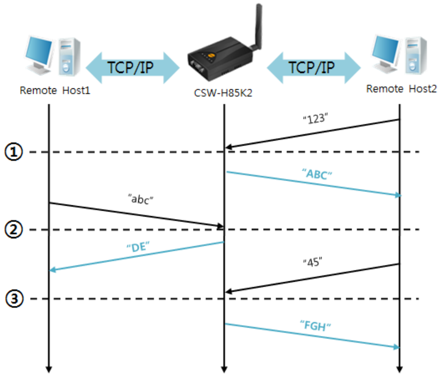
图 5-11 UDP动态HOST传送例
