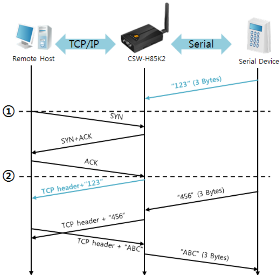
图 5-2 连接前数据大小为1的情况
