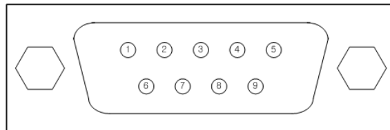
图 1-6 9针 D-sub female连接器
