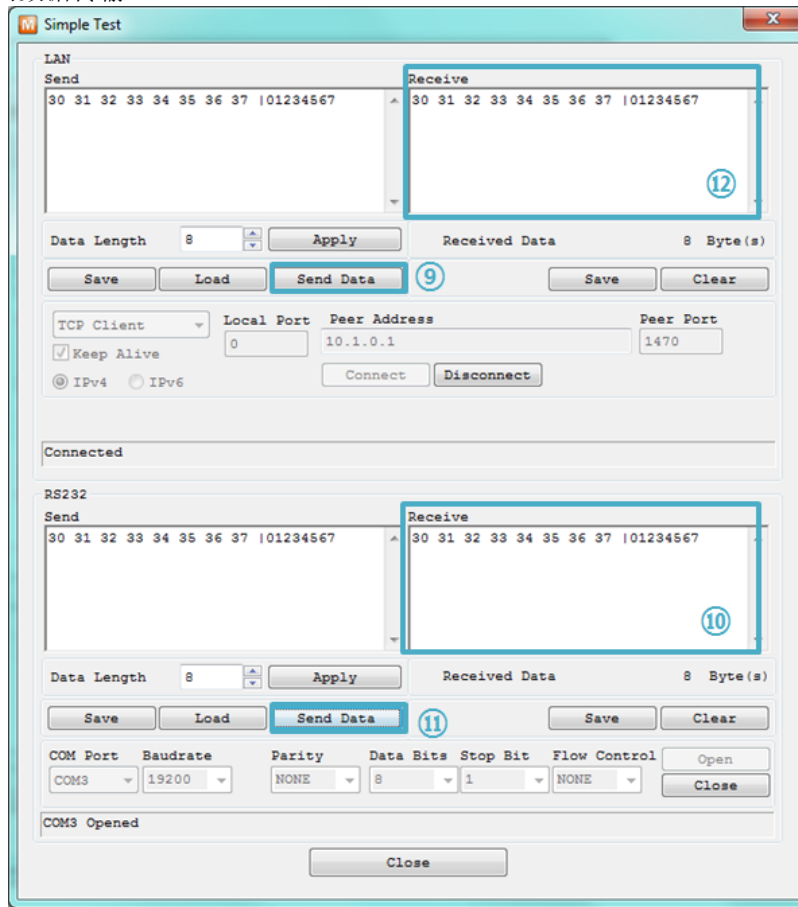
图 2-16 正常数据传送
