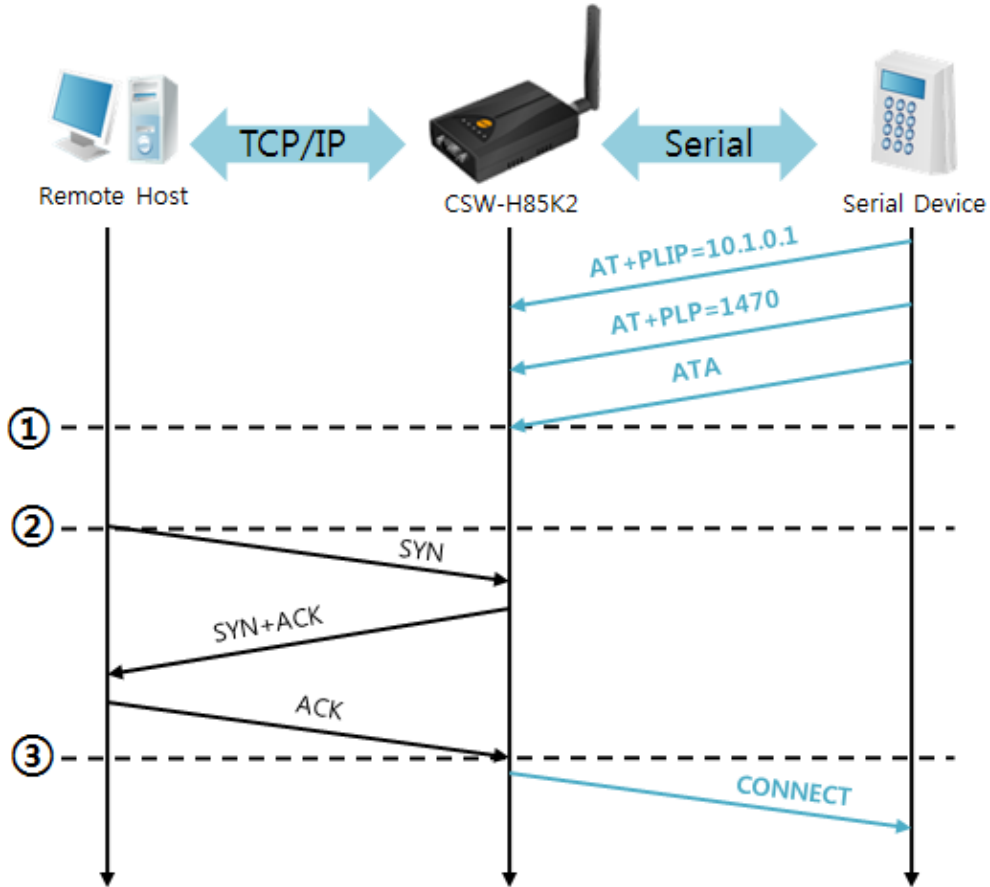
图 5-7 TCP 手动连接
