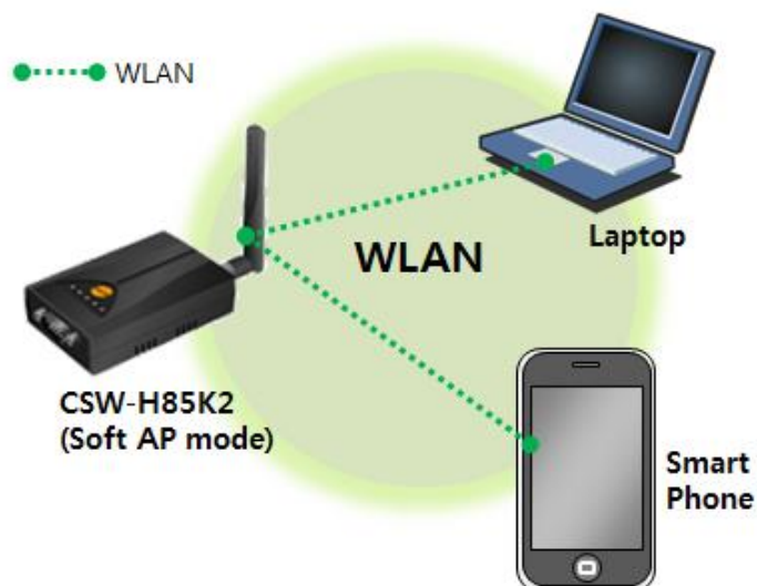
图 2-4 Soft AP 模式
