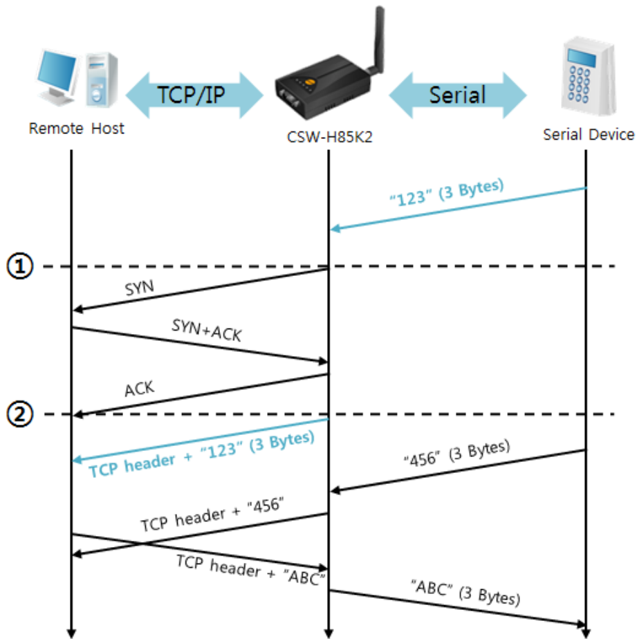
图 5-5 连接前数据大小为5的情况
