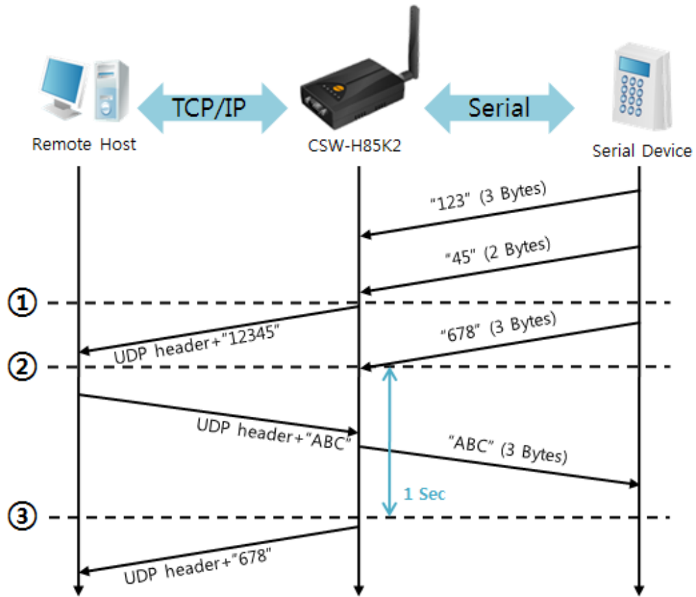
图 5-10 设定数据包 5, 数据帧间隔为100的情况
