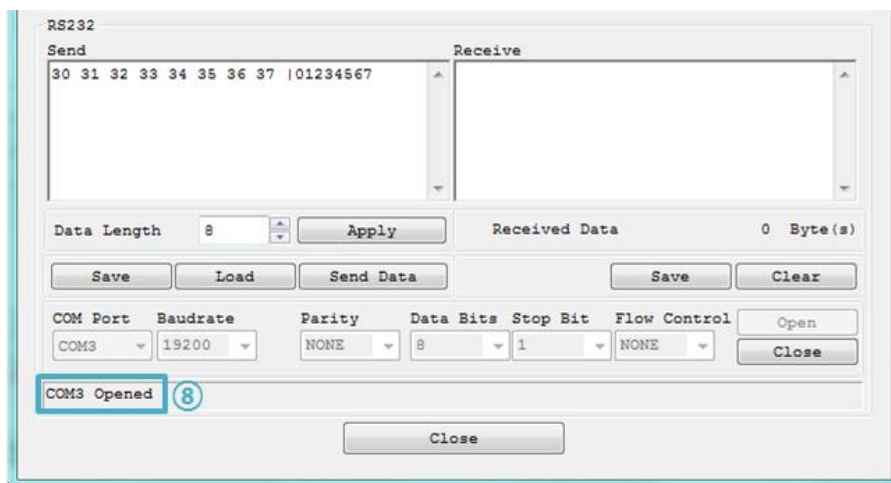
图 2-15 确认COM端口打开
