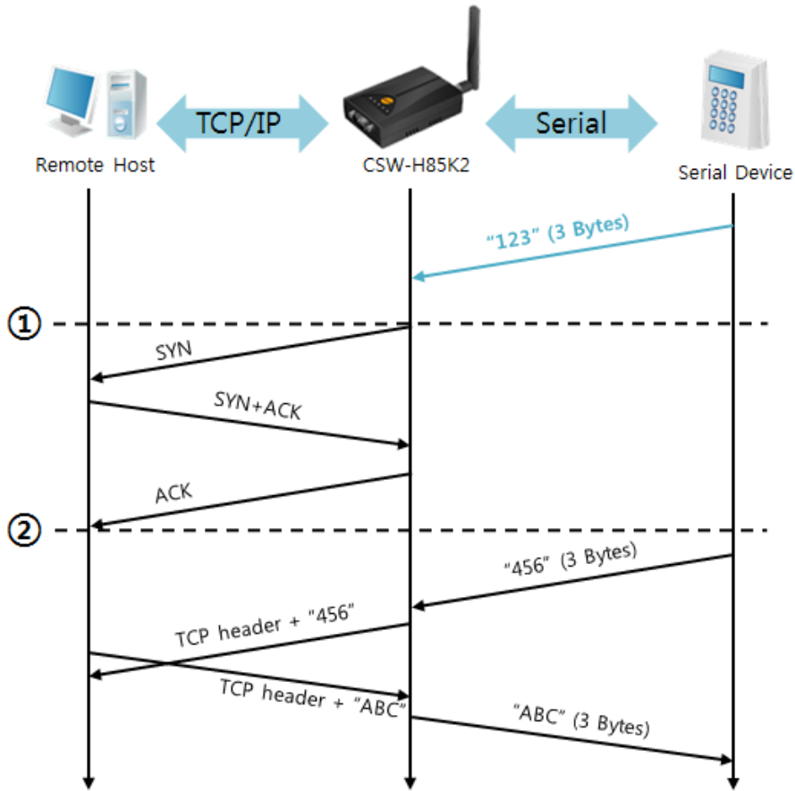
图 5-4 连接前数据大小为0的情况
