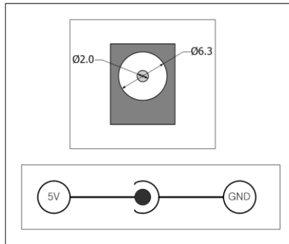
图 1-7 电源适配器
