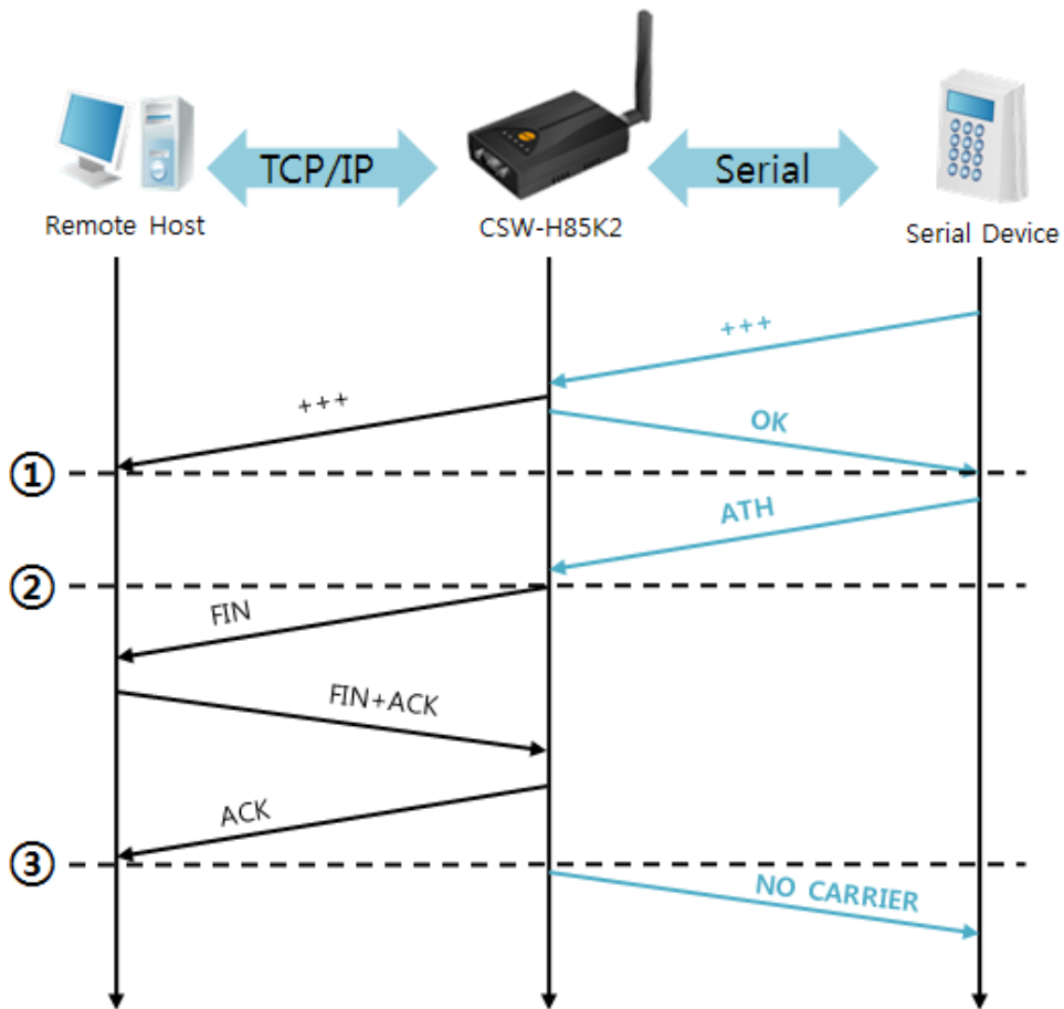
图 5-9 TCP 连接终止
