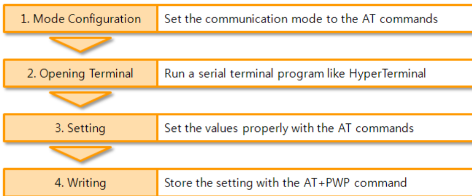
图 3-6 通过AT命令的顺序
