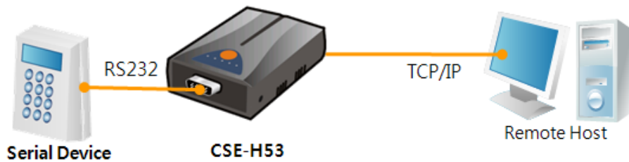
图 1-1 PC与 1:1连接
