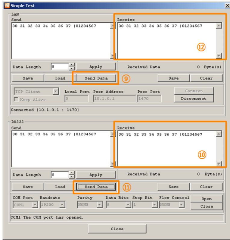
图 2-7 传送正常的的数据
