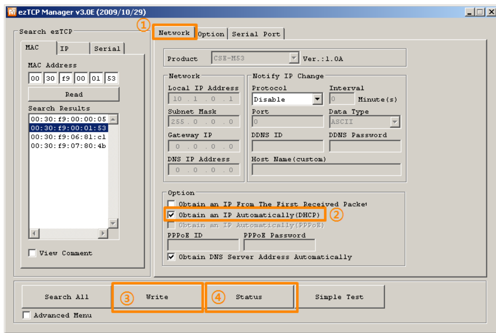
图 3-7 利用DHCP被分配IP地址
