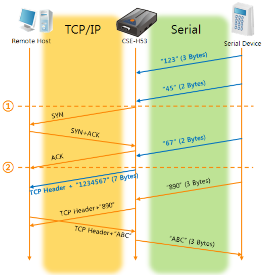
图 5-5 数据包设定为5的情况
