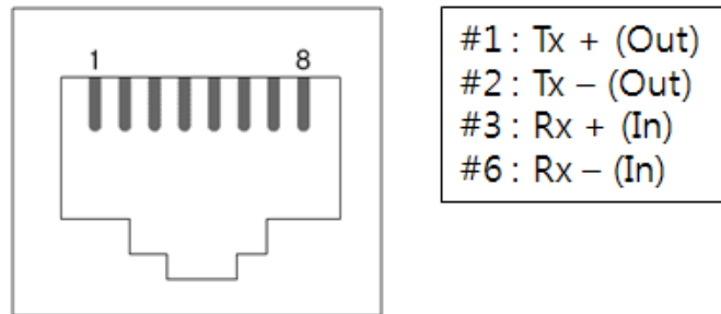
图 1-6 RJ45 以太网连接器规格
