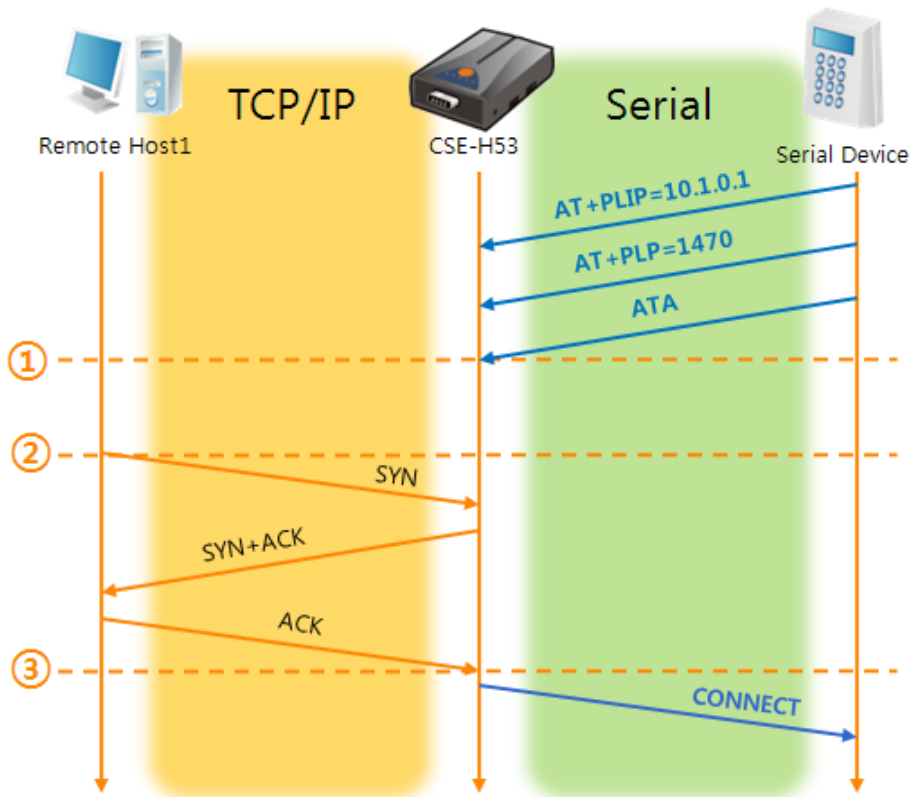
图 5-7 TCP 手动连接
