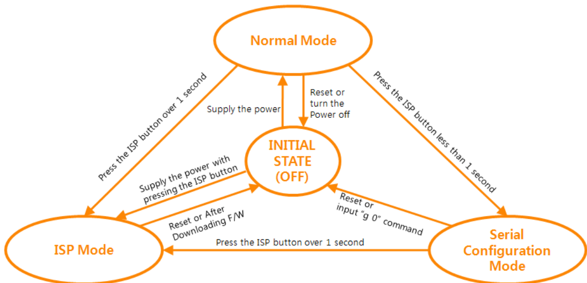
图 4-1 进入各动作模式方法
