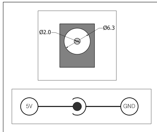
图 1-7 DC 5V 电源连接器
