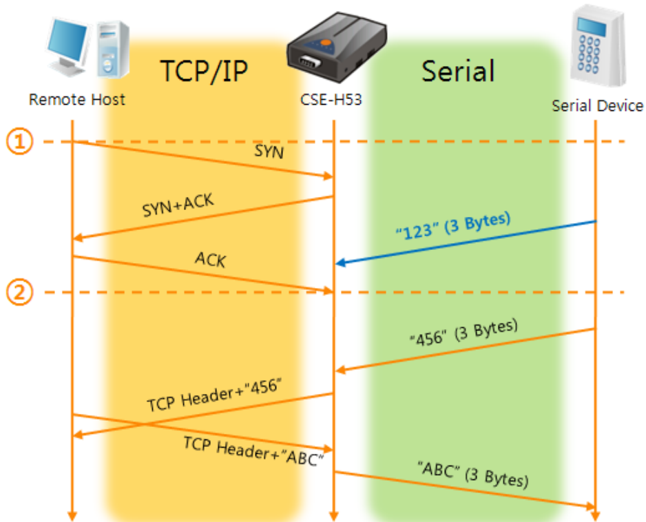
图 5-1 数据包设定为0时
