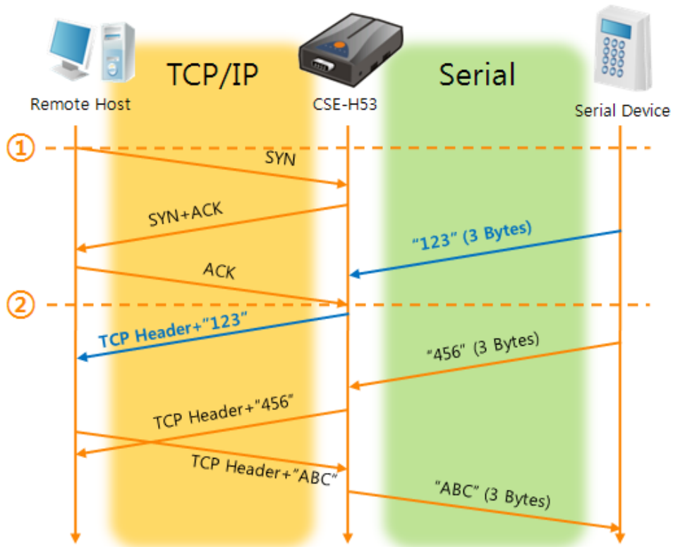
图 5-2 数据包设定为1的情况
