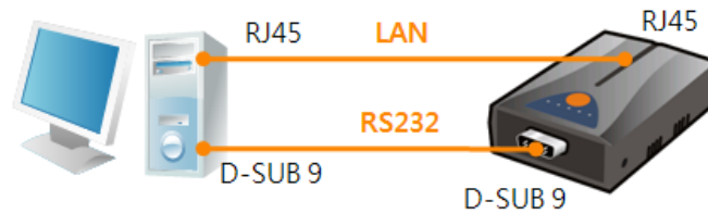
图 2-1 为了测试与PC连接
