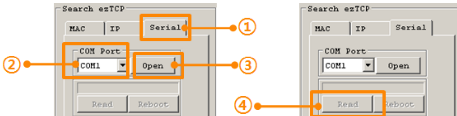
图 3-4 通过串行端口读取参数顺序
