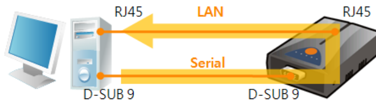
图 2-9 RS232 → LAN
