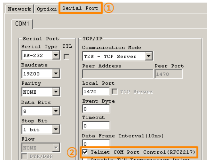
图 7-2 设定串行端口设定/传送状态功能시리얼
