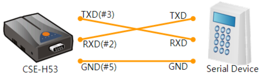
图 8-1 正确的RS232连接
