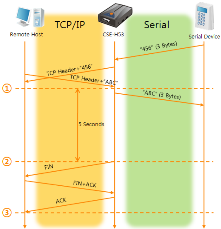
图 5-3 等待终止之间为5的时候
