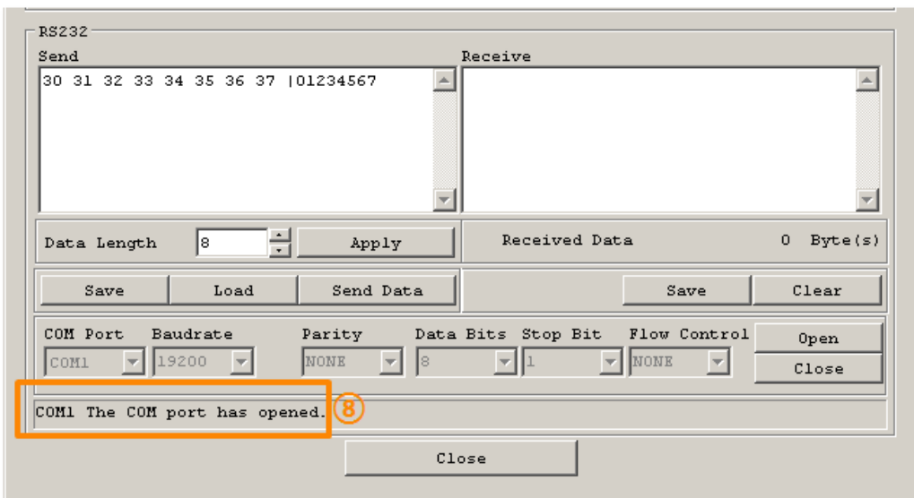
图 2-6 检查COM端口打开
