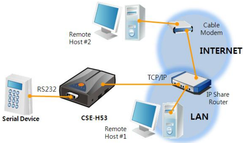
图 1-4 应用IP路由器的构成 例
