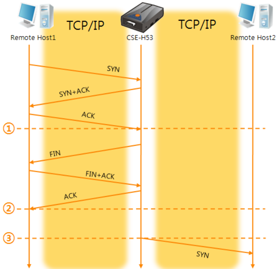
图 5-6 TCP 服务器/客户端模式的情况
