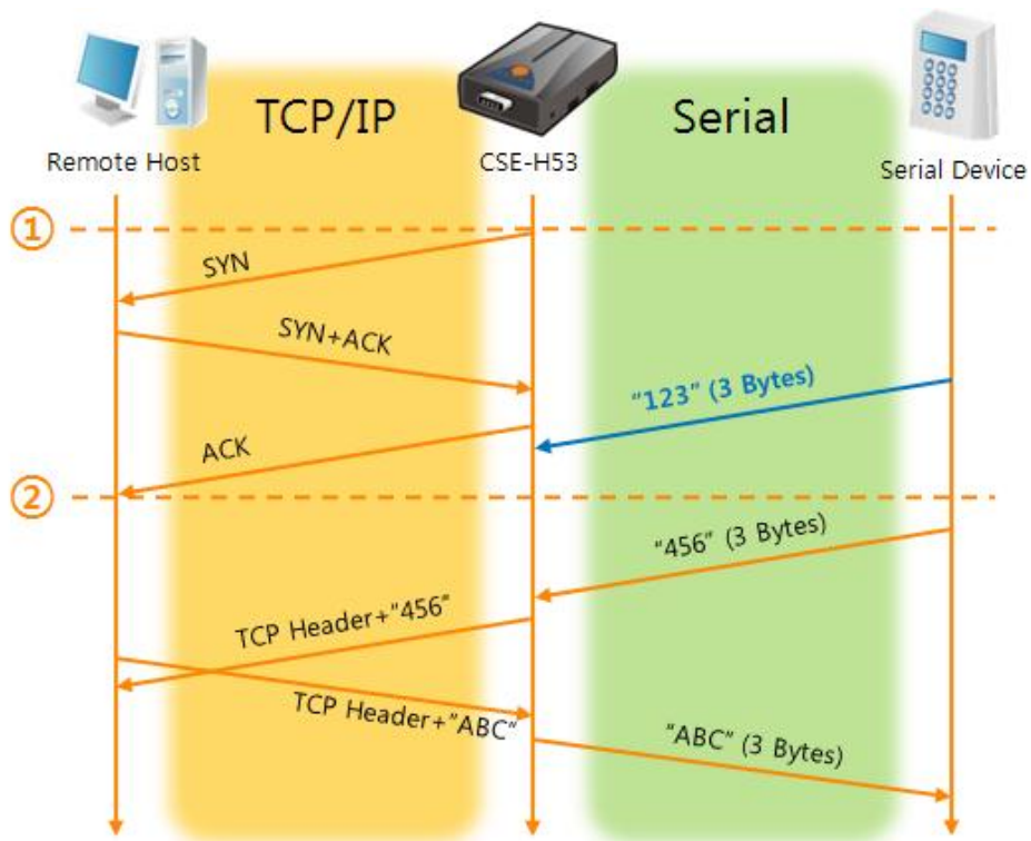
图 5-4 数据包设定为0的情况
