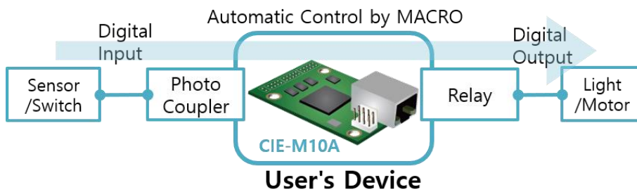
图 1-4 Macro模式使用构成例
