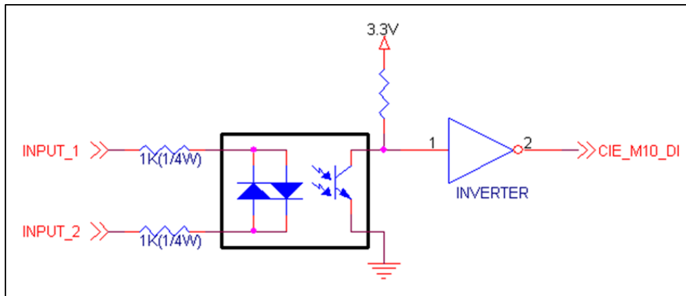
图 1-9 电压输入方式数字输入电路构成
