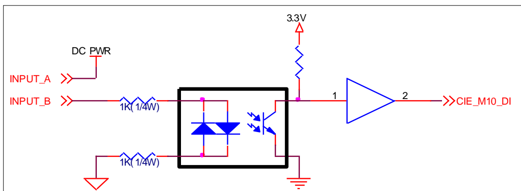
图 1-10 Dry-Contact方式数字输入电路图
