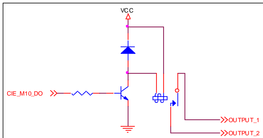
图 1-11 继电器接口电路图构成
