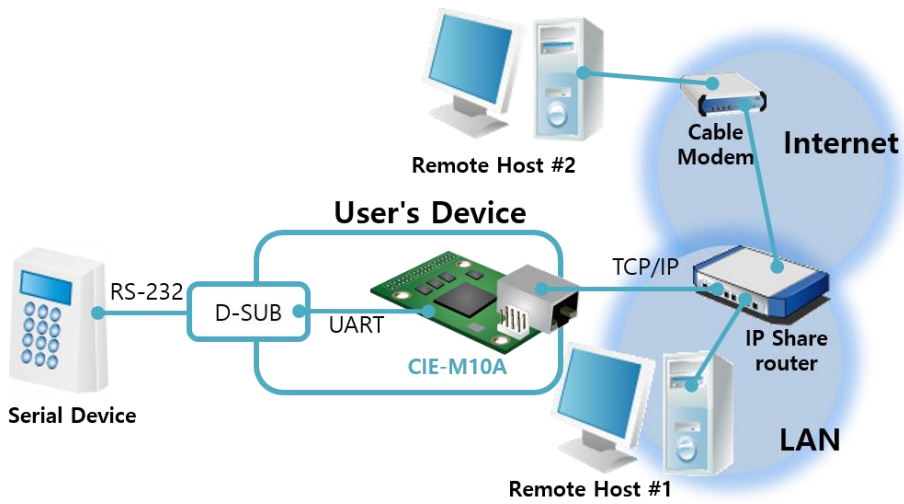
图 1-6 串行设备服务器构成 例
